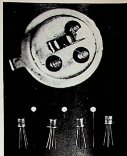
Afb. 7 UHF transistor AF139 (PNP) in vergelijking met spelden: hierboven een sterke vergroting.
